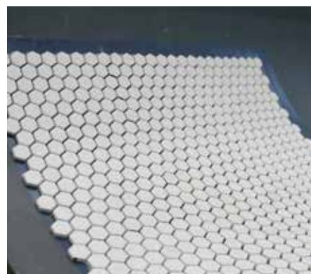
Carreaux d'alumine Belzona 9811 collés avec Belzona 1321
